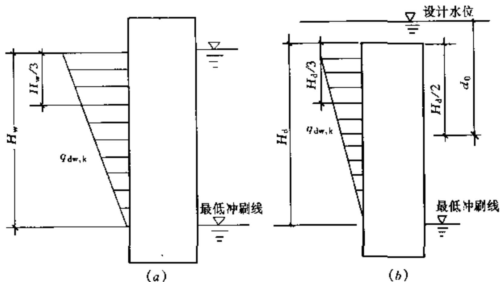
图 4.3.4 作用在取水头部上的流水压力图 (a) 非淹没式；(b) 淹没式
