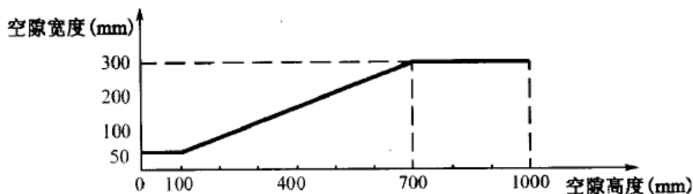
图 1 型钢间的空隙宽度的要求
